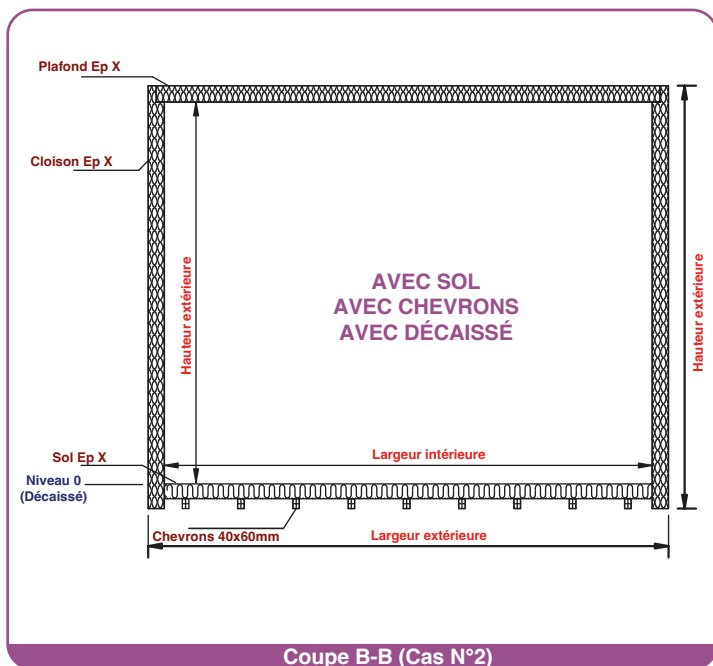
Coupe B-B (Cas N°2)
